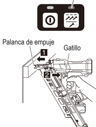
Indicador de operación de clavado (Iluminado en azul)
