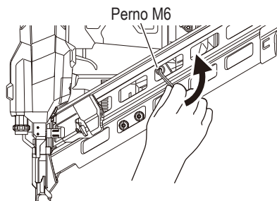
Perno M6
