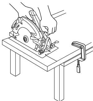
EXEMPLE TYPE DE SOUTIEN MANUEL DE LA SCIE ET, SOUTIEN LA PIÈCE ET D'ACHEMINEMENT DU CORDON.
