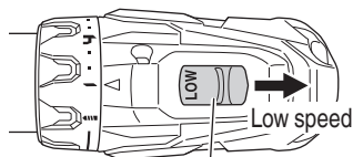
Shift knob
