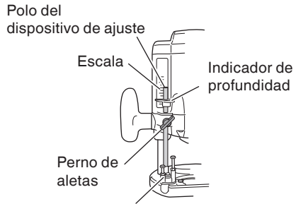
Bloque del dispositivo de ajuste
