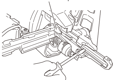
Cuchilla impulsora
